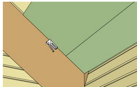
10. Ilmansulkukaistojen asennus palkkien alapintaan, limitys 200 mm.
